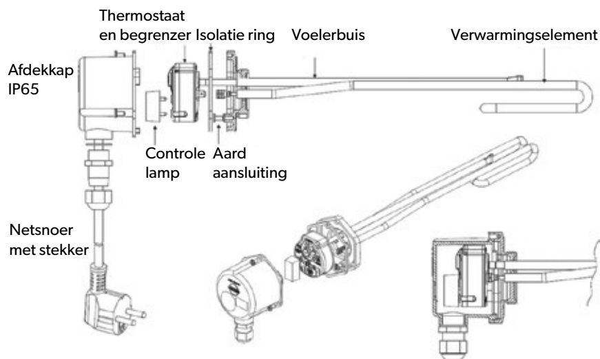
Figuur 9 Onderdelen van inschroefelement
