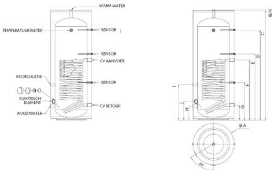
Figuur 1 Boiler verticaal t.b.v. warmtepomp
