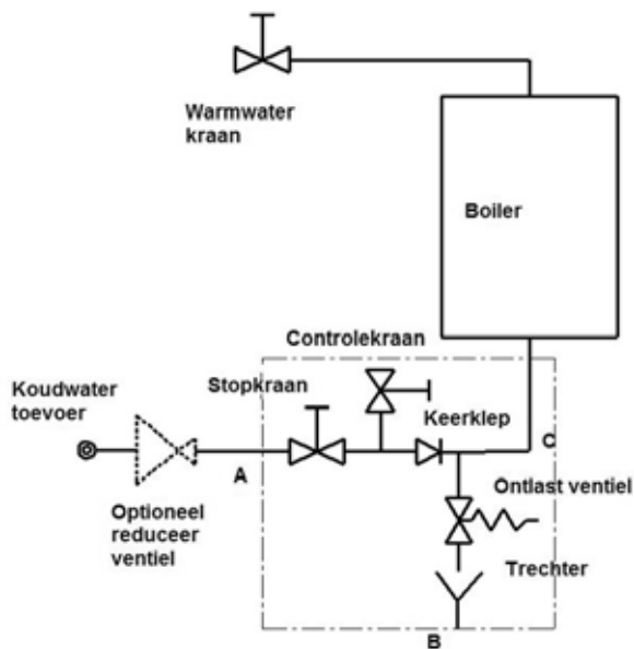
Figuur 5 Schema inlaatcombinatie
