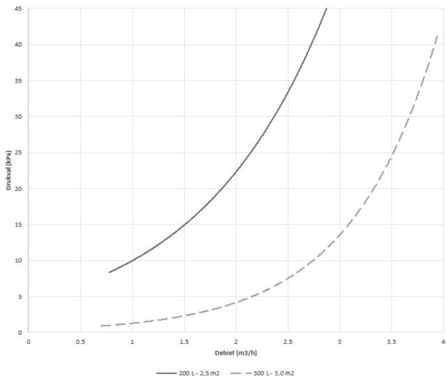
Figuur 2 Drukverlies warmtespiralen
